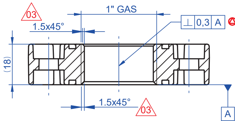
Sez. A-A
